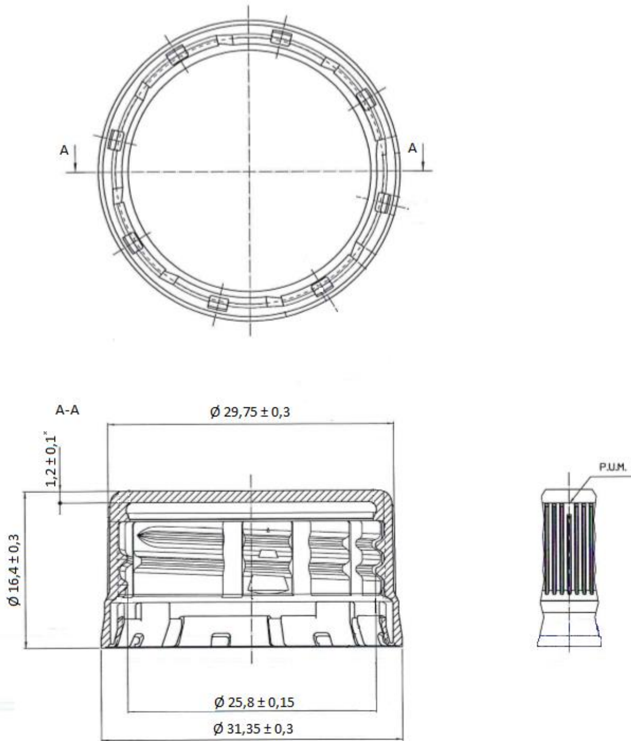
Рисунок А.05 – Колпачок Тип I-05 (ML 1881-120) по СТО 80272675-001-2016
