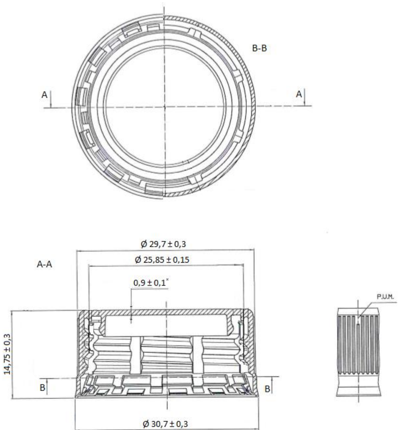
Рисунок А.07 – Колпачок Тип II-01 (АВ 1881-120К) по СТО 80272675-001-2016
